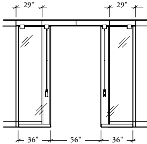
36" wide: 56" door clearance
