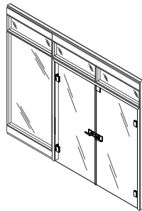
F D C Glass Barn Door
