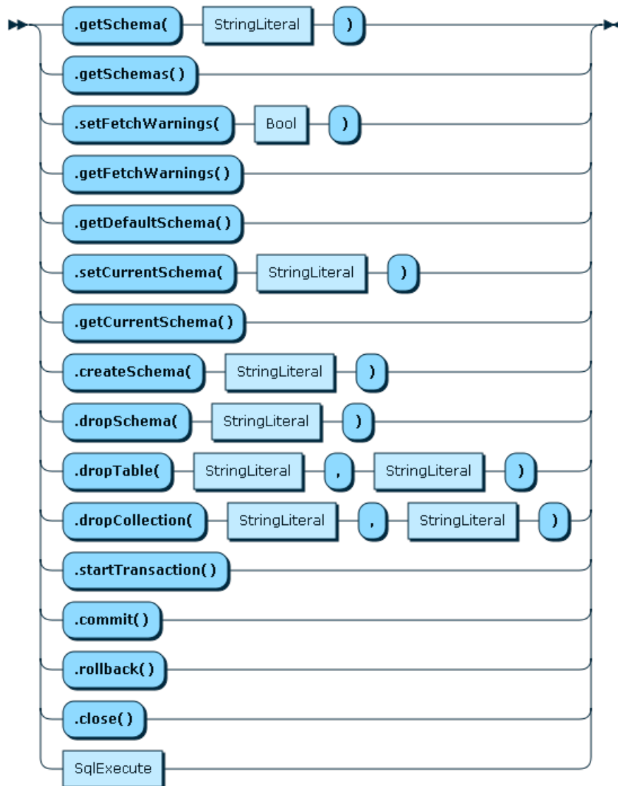
Figure 11.2 NodeSession
