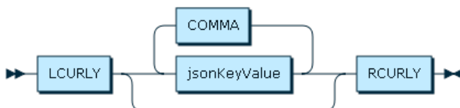
Figure 12.17 jsonDoc
