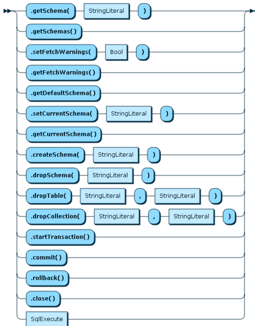
Figure 11.2 NodeSession
